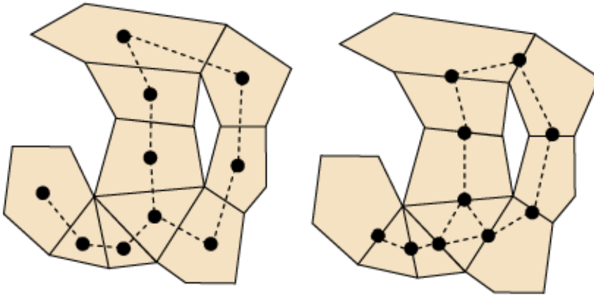
Figura 4. Ejemplo de una malla de navegación con los caminos usando los centros de los polígonos (izquierda) o las aristas (derecha)
