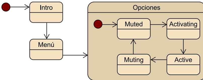
Figura 2. Ejemplo de un diagrama de estados con subestados
