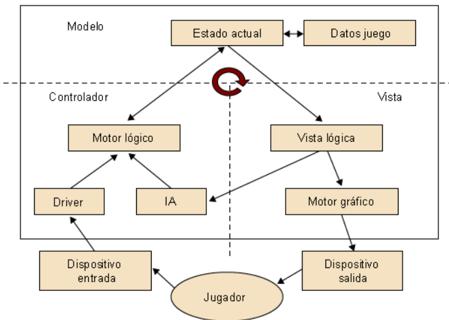
Figura 1. Esquema modelo-vista-controlador
